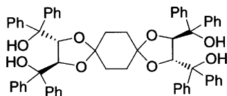
6 a: ( R,R,R,R )-(–)-form b: ( S,S,S,S )-(+)-form Chart 2.
